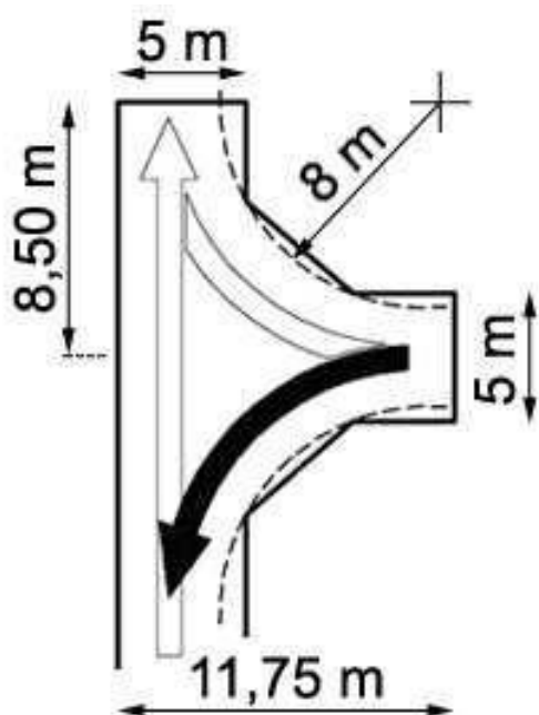
Aire de retournement en L
